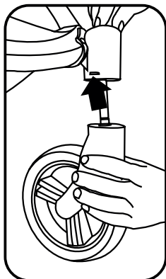
Ruchomy przycisk do wyjmowania koła
